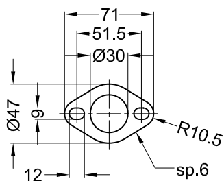
Vista "B" Flangia "43D"
