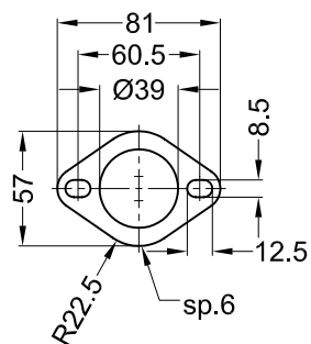
Vista "B"
