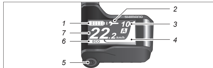
Abb. Display SC-EM800
