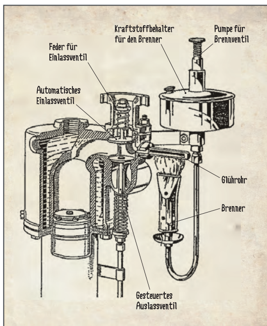
Bild 2: Motor mit Glührohrzündung
