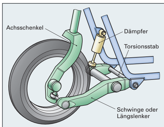
Bild 2: Achsschenkellenkung
