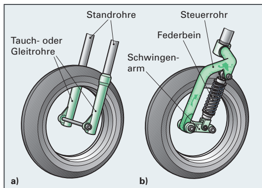
Bild 3: Vorderradführung
