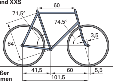
Rahmengeometrie für Renn- und Sporträder in XXL und XXS
