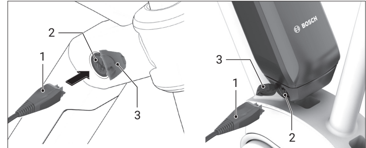
Abb.: 13 Laden des Akkus am E-Rad
