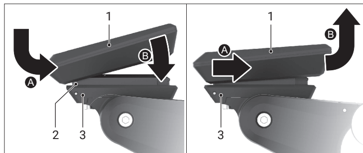
Afb.: 22 Montage bedieningscomputer Kiox 300
