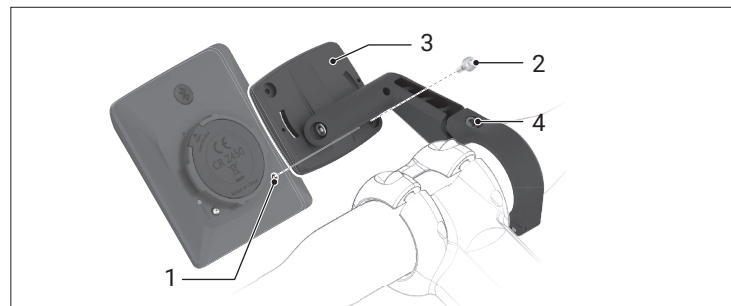
Afb.: 29 Plaatsen van de vergrendelingsschroef
