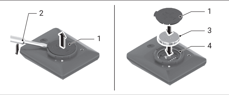
Afb.: 30 Plaatsen van de vergrendelingsschroef
