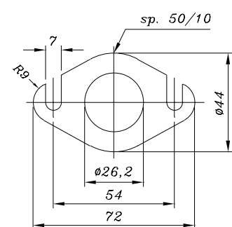
Vista da "A" Flangia tipo "99A"
