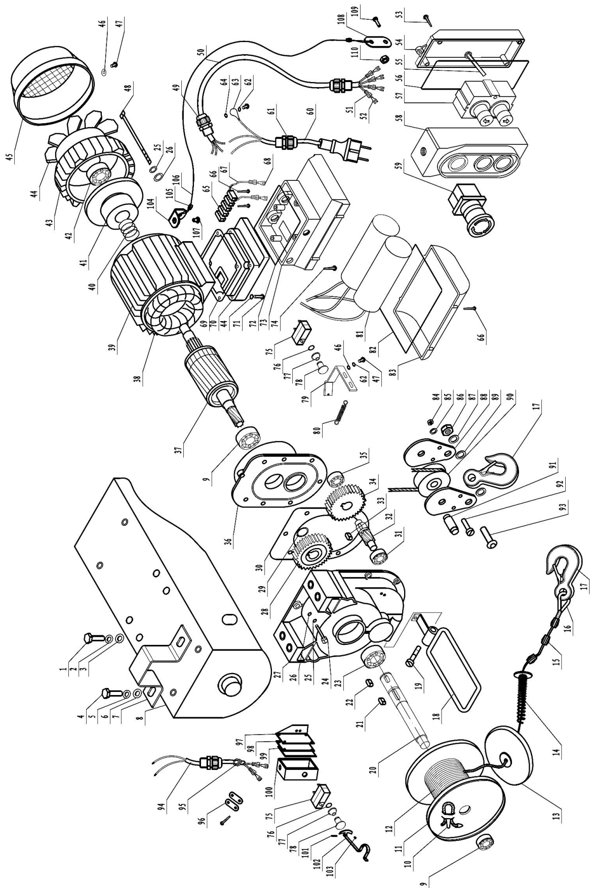
Abb. / Fig. 3: Ersatzteilzeichnung - MES 999-2 / Spare parts drawing - MES 999-2
