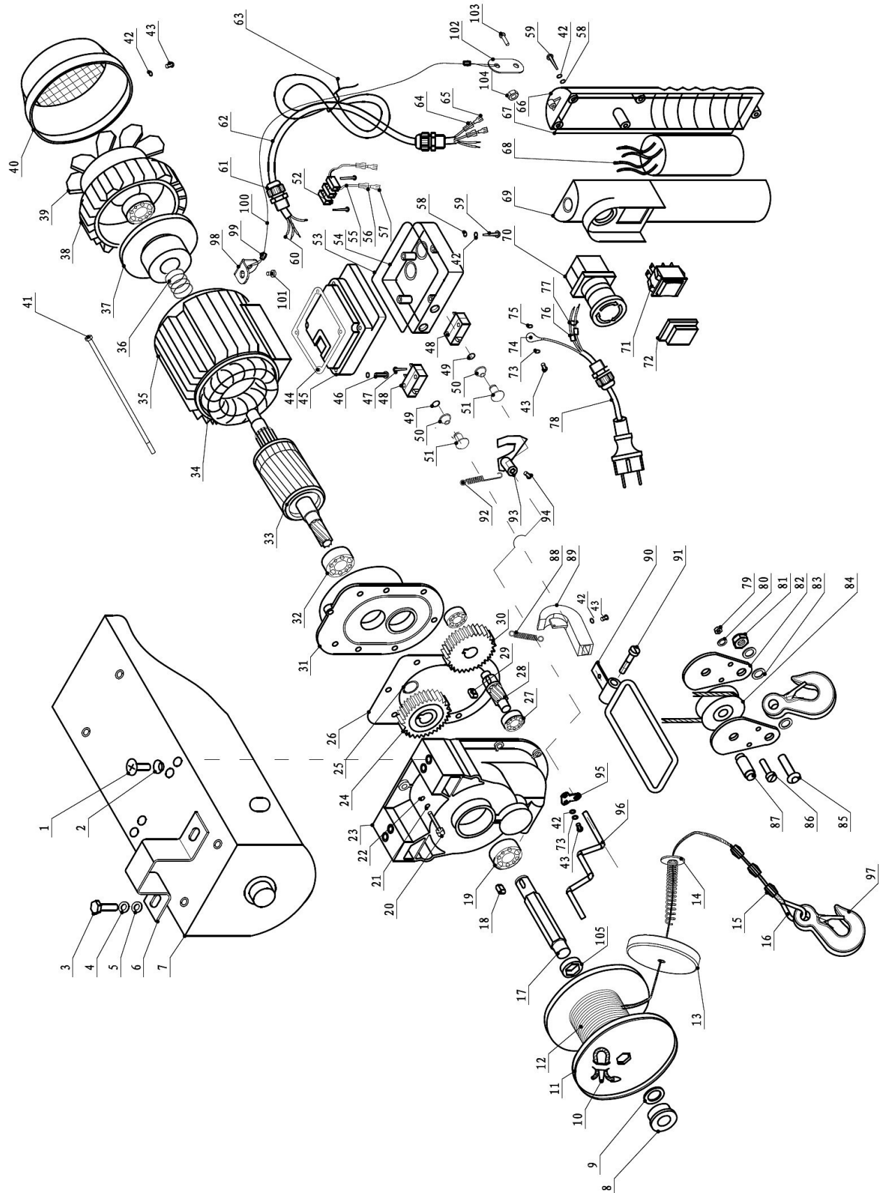
Abb. / Fig. 2: Ersatzteilzeichnung - MES 600-2 / Spare parts drawing - MES 600-2
