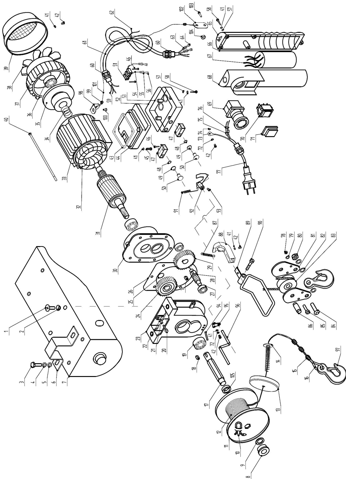
Abb. / Fig. 1: Ersatzteilzeichnung - MES 250-2 / Spare parts drawing - & MES 250-2
